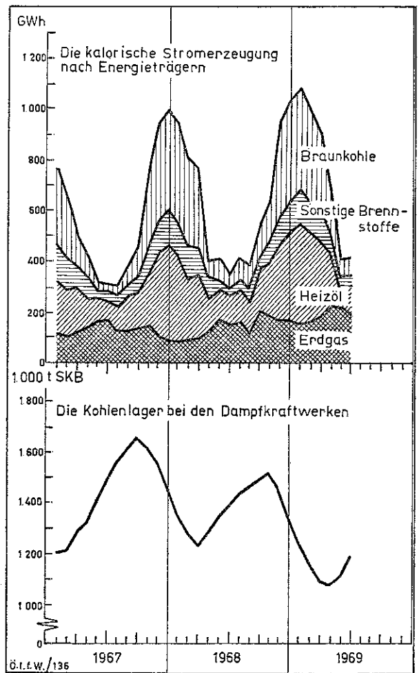
Die kalorische Stromerzeugung nach Energieträgern
